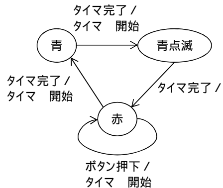
付図 1．歩行者用信号の状態遷移図
