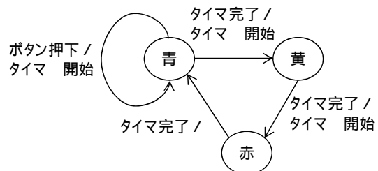
付図 2．車道用信号の状態遷移図
